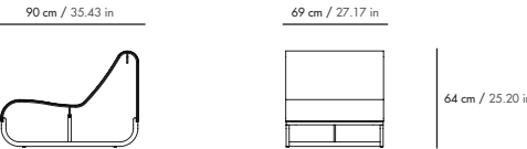
Module central / Central module EM3TCM
