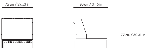
Module central pouf / Ottoman central module EM18SCP
